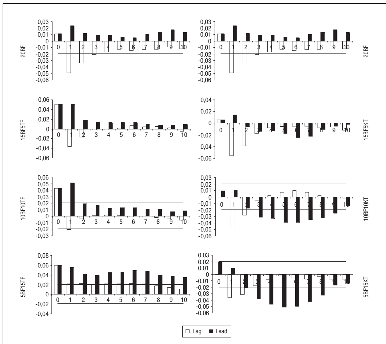
Figura 2 Correlaciones cruzadas del rendimiento con el volumen para combinaciones de BF y TF (izquierda) y BF y KT (derecha) (Pt, Vt-i) lags, (Pt, Vt+i) leads
