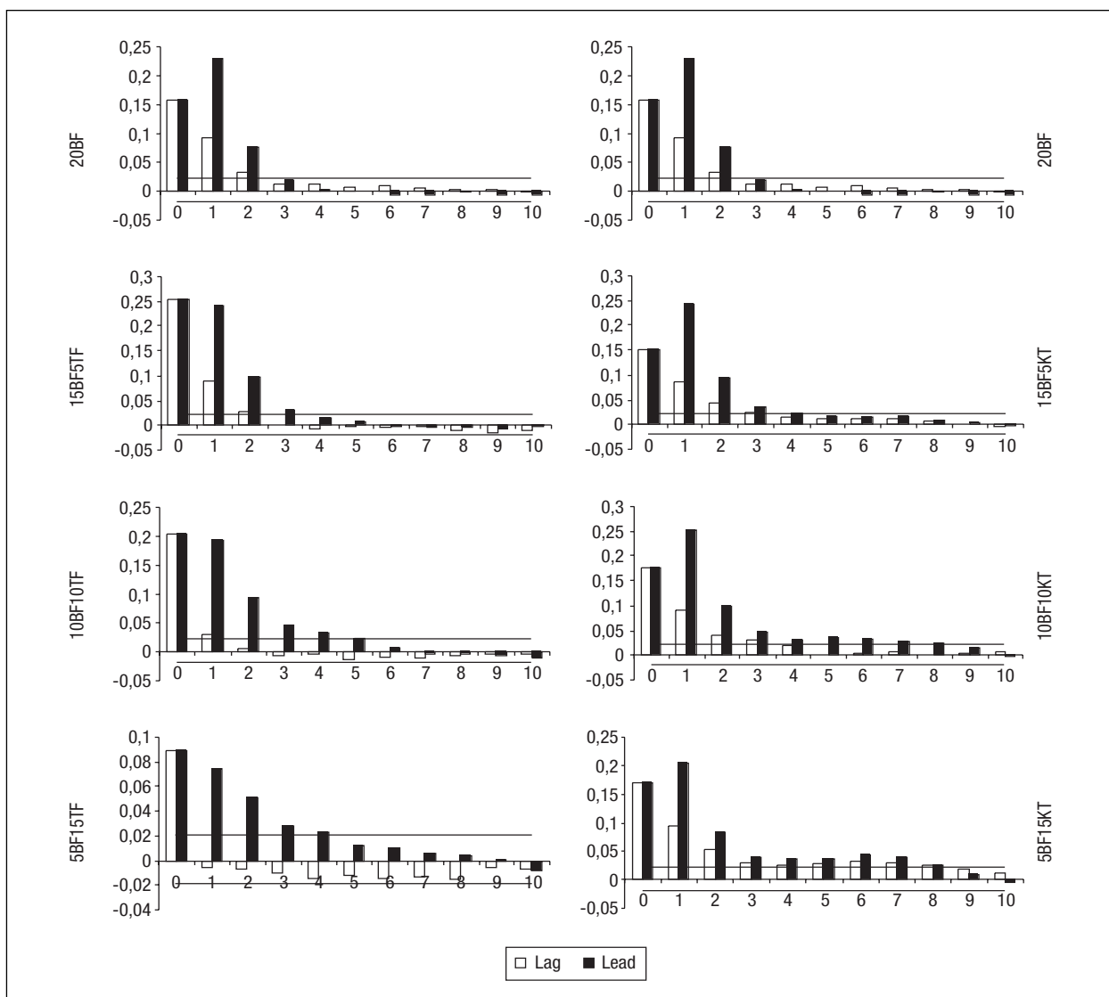
Figura 3 Correlaciones cruzadas de la velocidad con el volumen para combinaciones de BF y TF (izquierda) y BF y KT (derecha) (Pt, Vt-i) lags, (Pt, Vt+i) leads
