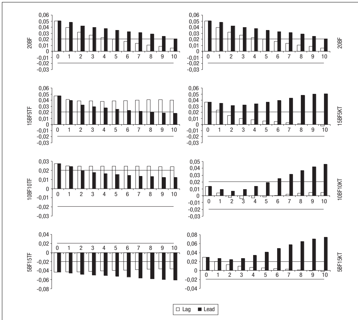
Figura 1 Correlaciones cruzadas del precio con el volumen para combinaciones de BF y TF (izquierda) y BF y KT (derecha) (Pt, Vt-i) lags, (Pt, Vt+i) leads
